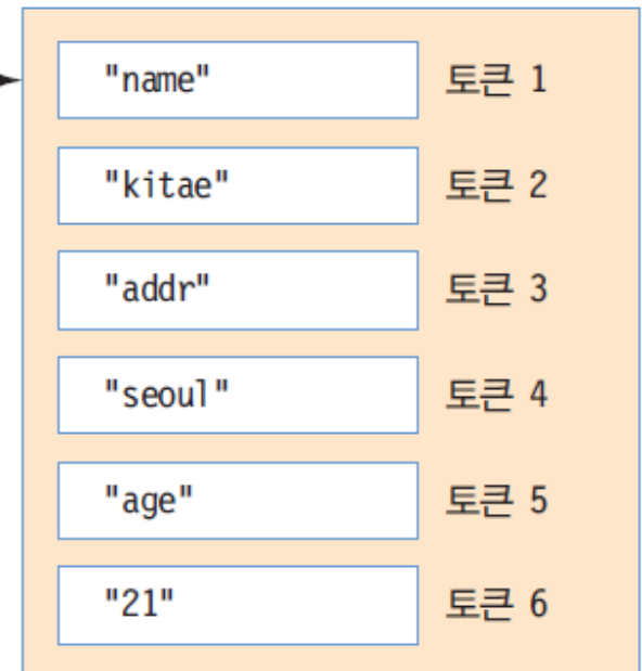
StringTokenizer 객체
