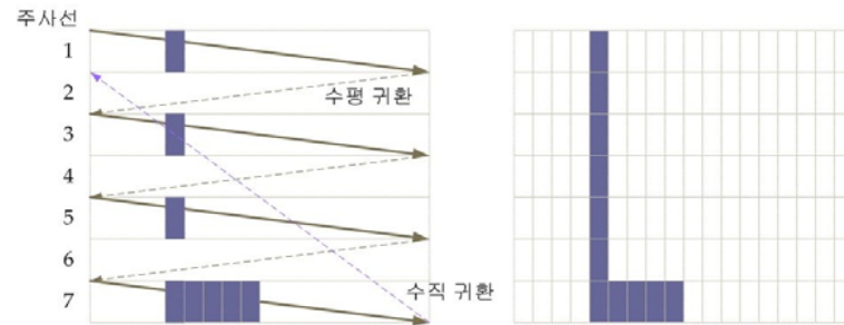
래스터 영상, 화소, 주사선 사이의 관계
