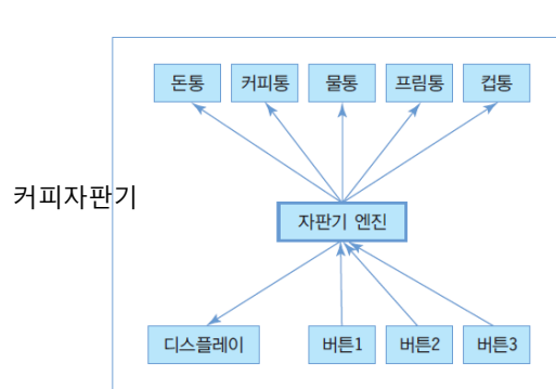
객체지향적 프로그래밍의 객체들의 상호 관련성
