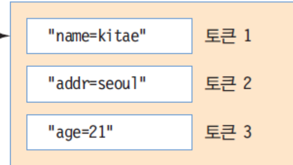
StringTokenizer 객체
