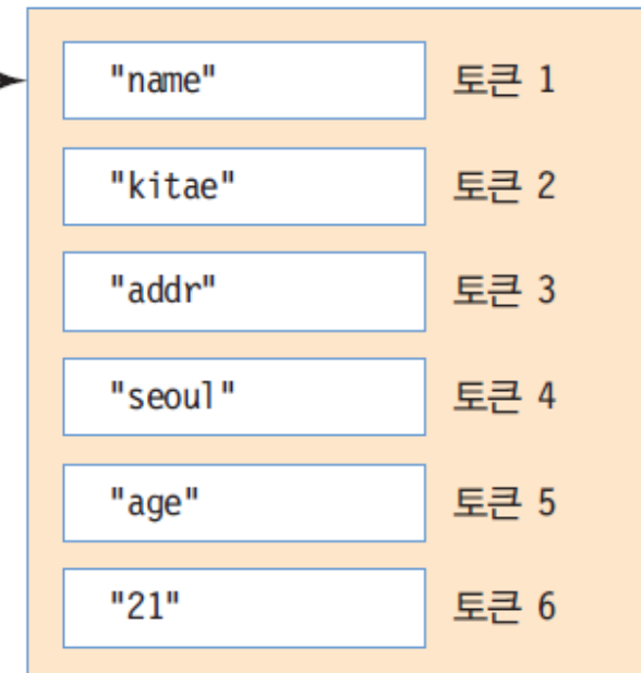
StringTokenizer 객체
